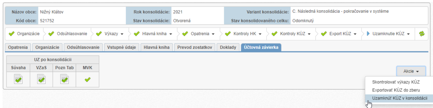
Obrázok 17: Uzamknutie KÚZ
