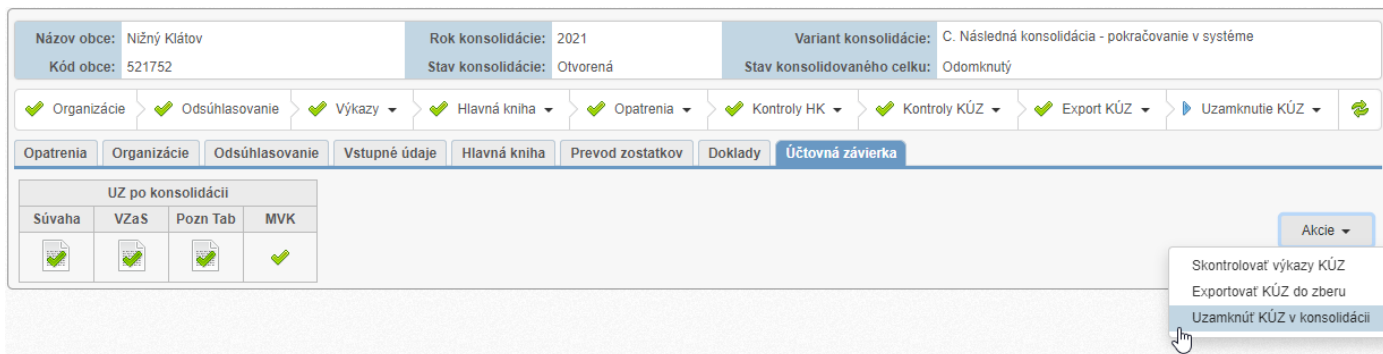
Obrázok 129: Uzamknutie konsolidácie
